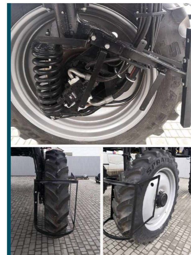
Ілюстрація монтажу каркаса захисних розсікачів
